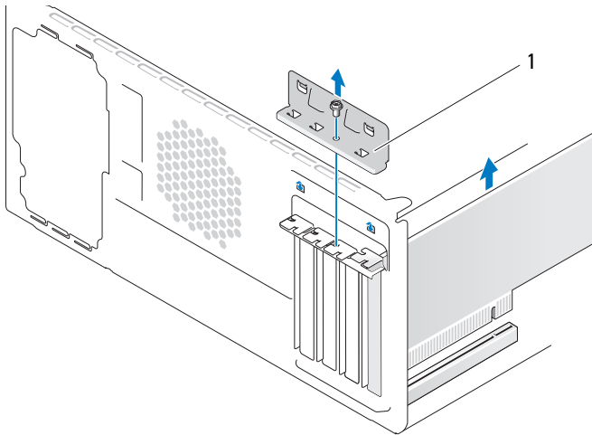
1 Soporte de retención de la tarjeta
