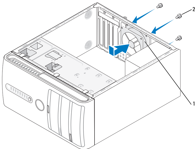
1 Ventilador del chasis 2 Tornillos (4)
